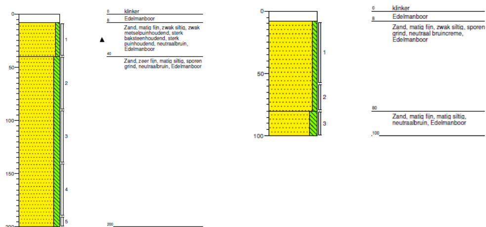
Afbeelding 5: boorprofielen boring 301 (links) en boring 308 (rechts, Buro Ontwerp & Omgeving)
