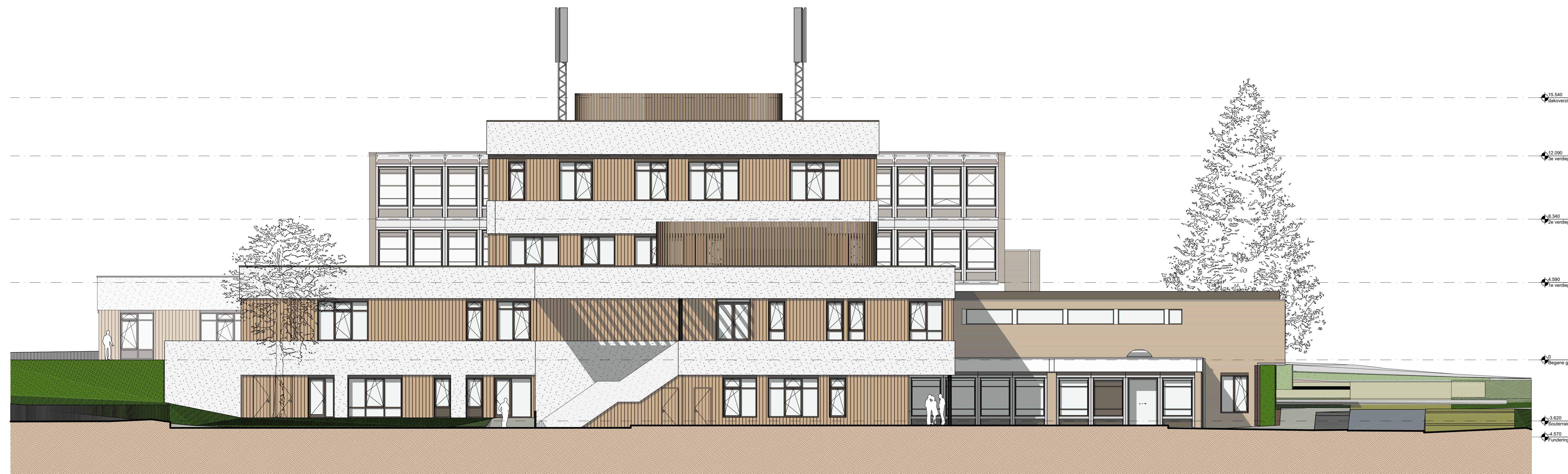
Linkergevel - 1:100
