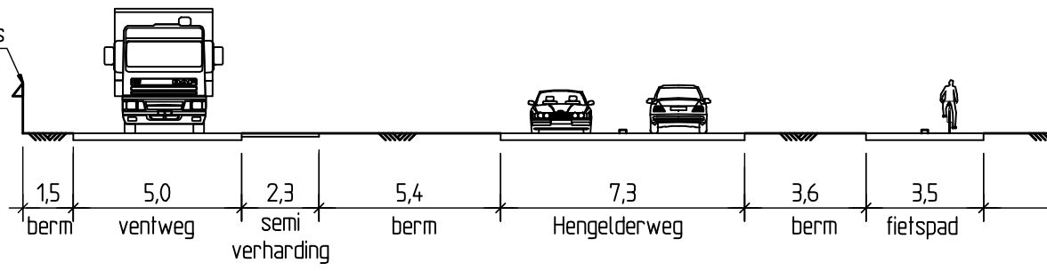
Dwarsprofiel A-A: Hengelderweg Schaal 1:200
